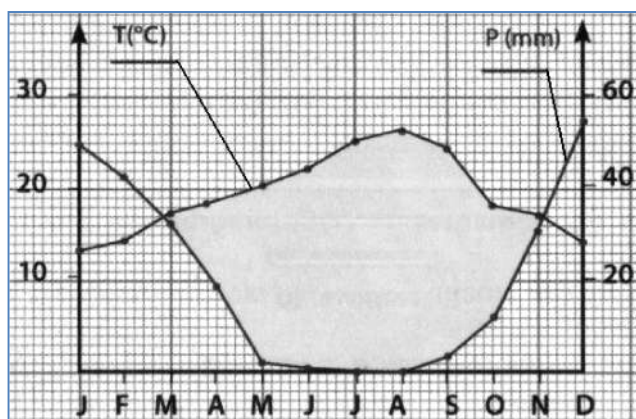
Figure 1 : diagramme ombrothermique de la station B.
